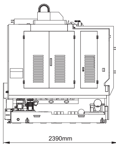
左视图
