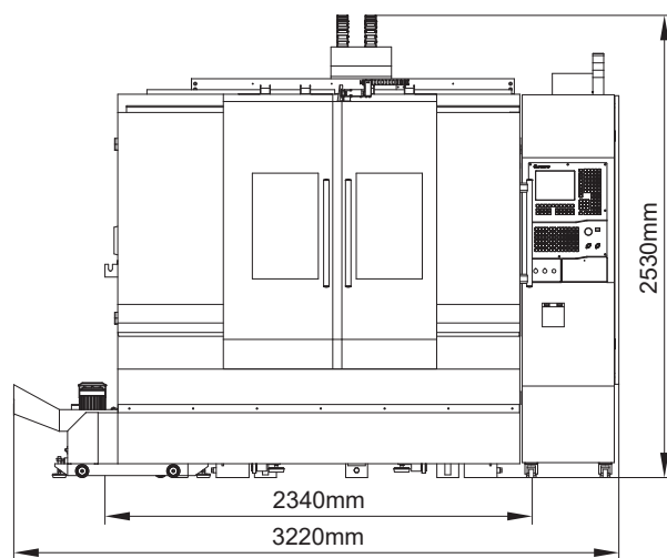
前视图
